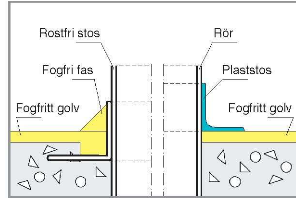
Anslutning av rostfri respektive plaststos kring rörgenomföring i betonggolvet.
