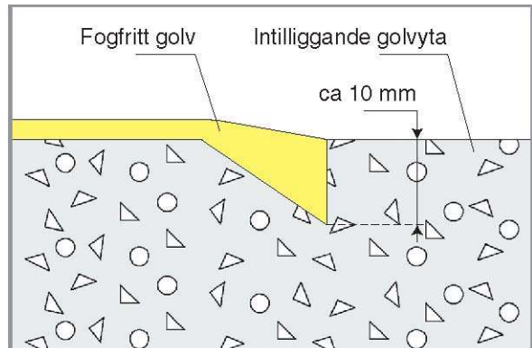
Vid anslutningar mitt på golv utförs en ursparing så att en jämnare övergång och förstärkning erhålls.
