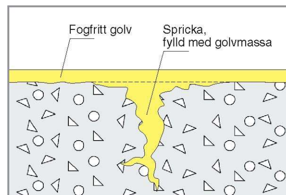
I förekommande fall rekommenderar produktleverantören, att spackling utförs och ett heltäckande fogfritt golv läggs över sprickor . I speciella fall, med vida sprickor , utförs sågning igenom golvet och fogning görs i spår.
