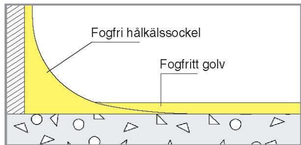
Hålkälssockel : höjd 50-200 mm, radie 30 mm. Hålkälssockeln applicerad före golvbeläggningen.
