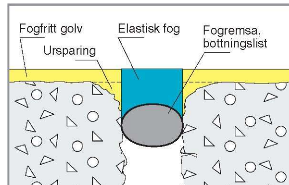
Vid befintlig dilatationsfog/spricka kan anslutning med elastisk fog göras synlig (se även sprickor).
