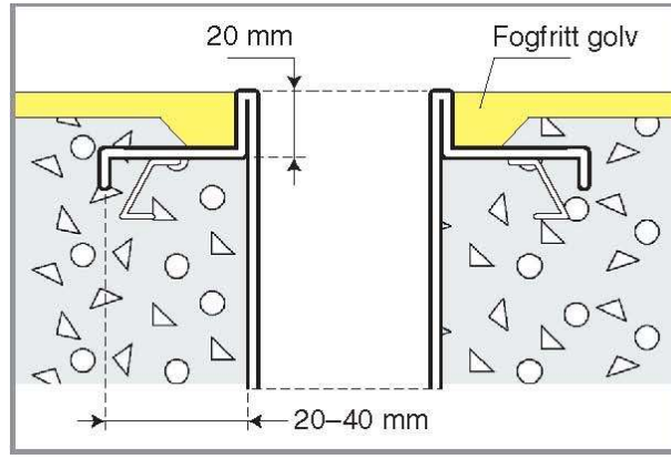
Anslutning vid rostfria brunnar, rännor och fettavskiljare.
