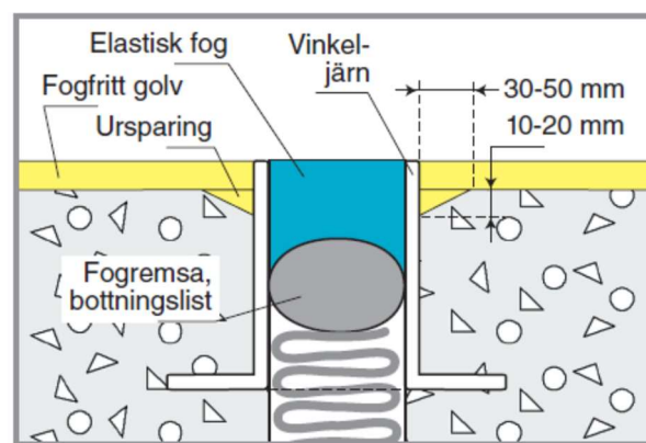
Anslutning till ny och befintlig expansions-/dilatationsfog utförs med en triangulär ursparing mot gods. Den elastiska fogmassan ska vara lika bred som djup och läggs på ett tätt bottningsmaterial.
