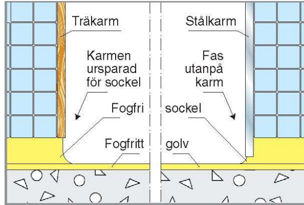
Ursparad respektive utanpåliggande anslutning runt dörrkarm mellan våtrummen.
