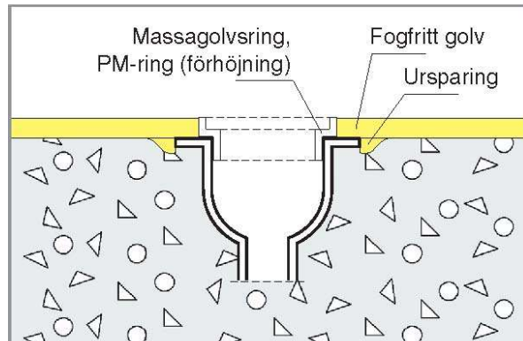
PM-ring används vid befintliga brunnar som förhöjning , t.ex. vid byte av ytbeläggning från plastmatta.
